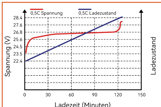
Ladezustandkurve (0,5C, 25°C)
