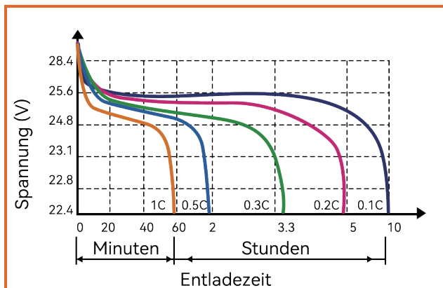
Entladecharakteristik (25°C)
